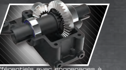
Différentiel avec engrenages à anneaux et pignons en acier Diferenciales con coronas dónicas y engranajes de pinones de acero Differentialien mit Stahling-Zahnrad und Ritzel
